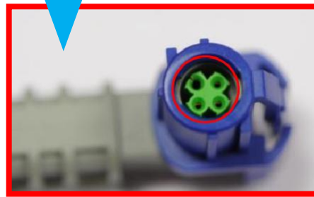
Abbildung 8-9 Beispiel: HSDe-Stecker
