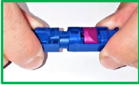
Abbildung 6-13 Richtiger Steckvorgang (Bsp. HSD)
