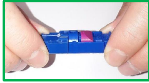
Abbildung 6-14 Richtiger Steckvorgang (Bsp. HSD)
