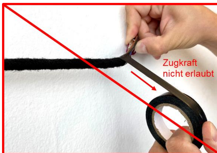
Abbildung 5-7 Falsches Abtrennen Klebeband
