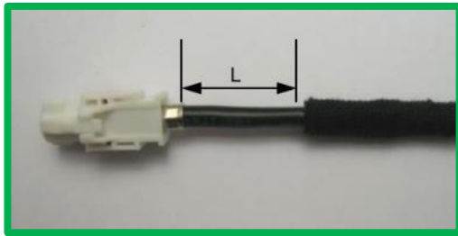
Abbildung 5-1 Bandagierte Einzelleitung (Bsp. HSD)
